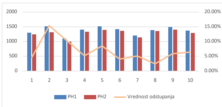
Slika 5: Uporedni prikaz vrednosti dve proždrljive heuristike i predstavljene u ovom radu za skup primera I2
