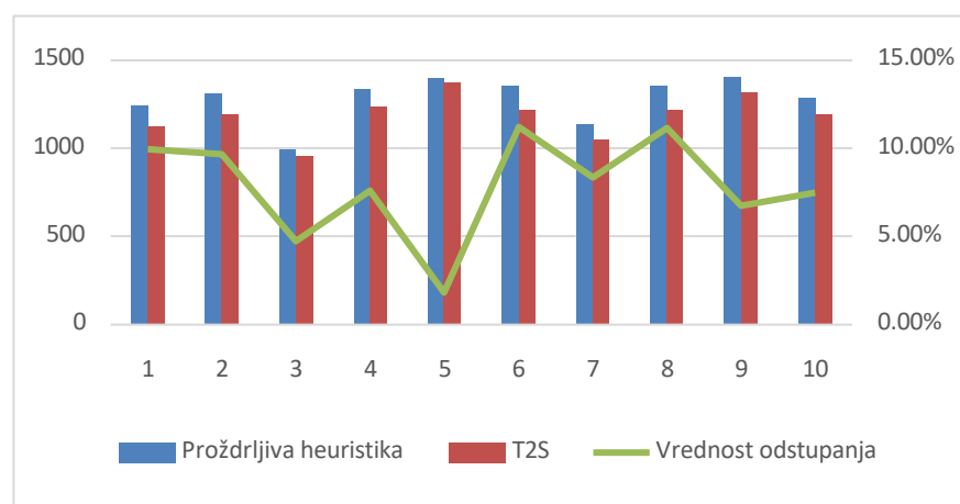
Slika 4: Uporedni prikaz vrednosti proždrljivog algoritma i tabu pretraživanja
