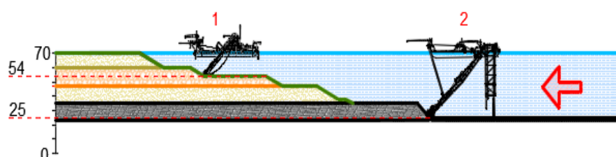
Slika 1: Podvodna eksploatacija uglja i pratećih sedimenata na Rudniku Kovin (Rudarski institut Beograd)
