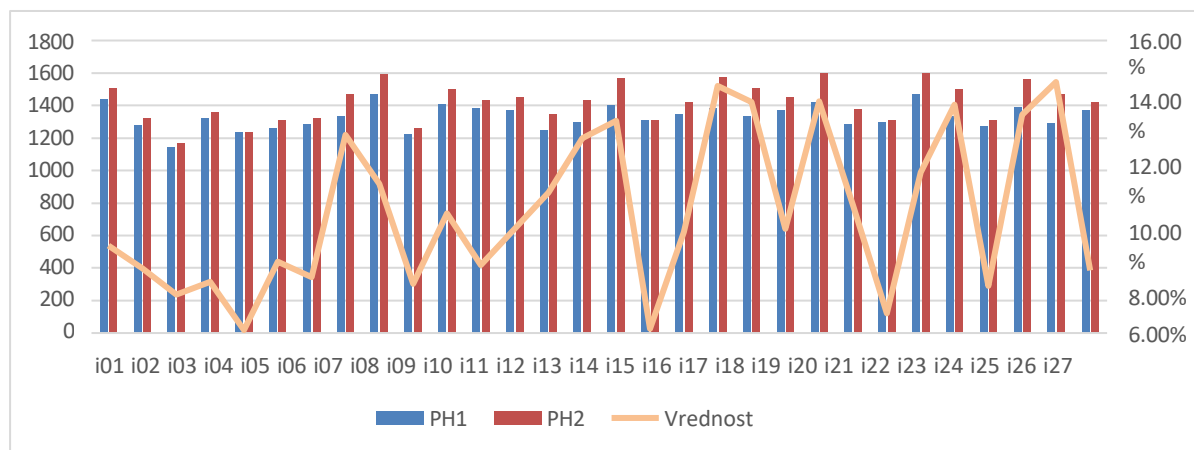
Slika 6: Uporedni prikaz vrednosti dve proždrljive heuristike i predstavljene u ovom radu za skup primera I3
