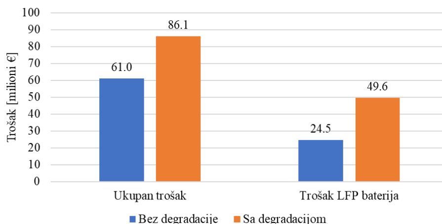
Slika 2. Ukupni troškovi implementacije e-autobusa (levo) i troškovi nabavke LFP baterija u posmatranom periodu (desno) sa i bez uračunavanja troškova degradacije baterija
