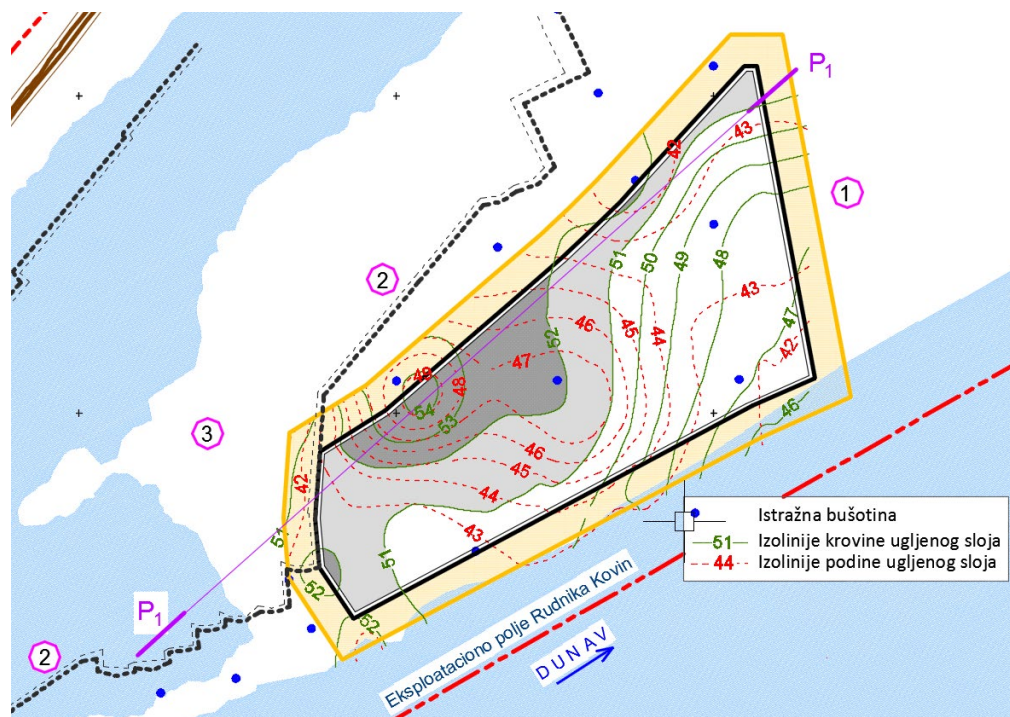
Slika 3: Model kovinskog ležišta uglja, u konturi eksploatacionog polja Rudnika Kovin, osnova sa izolinijama krovine i podine ugljenog sloja
