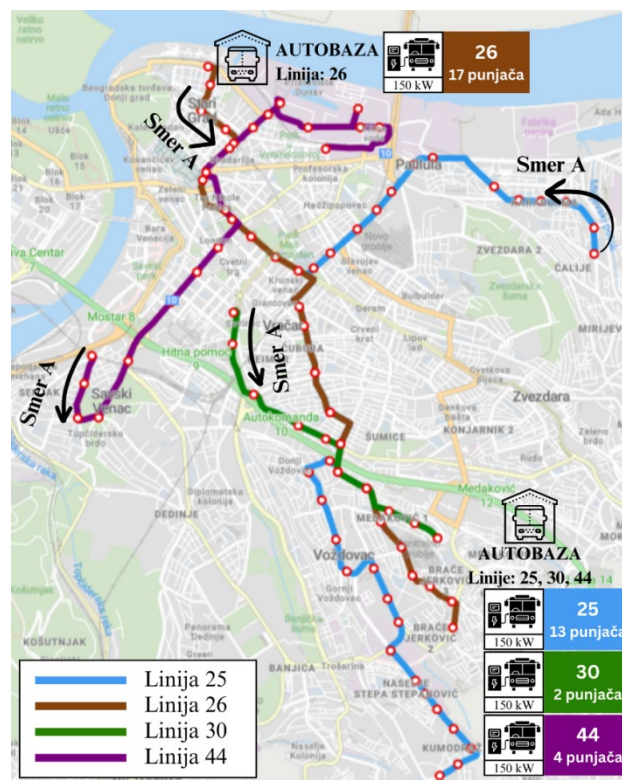
Slika 1. Prikaz razmatranih linija, pripadajućih autobaza i broj punjača koji se u njima nalaze
