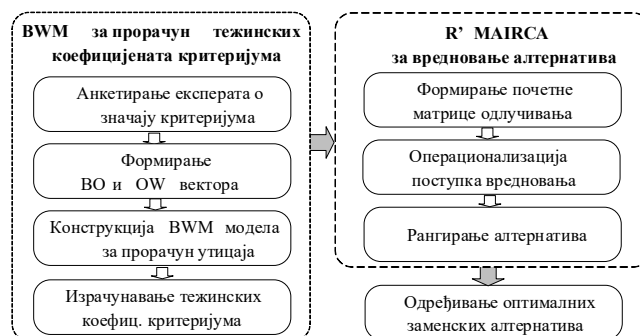
Слика 1: Хибридни BWM-R'MAIRCA модел
