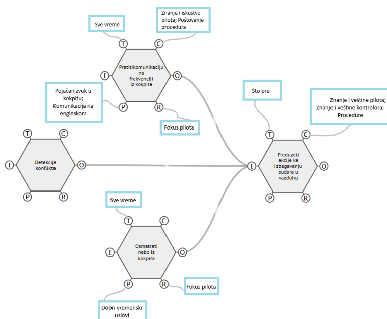
Slika 2: Vizuelni prikaz funkcija FRAM modela sudara
