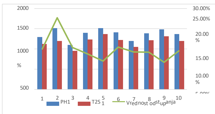
Slika 3: Uporedni prikaz vrednosti Proždrljivog algoritma i Tabu pretraživanja
